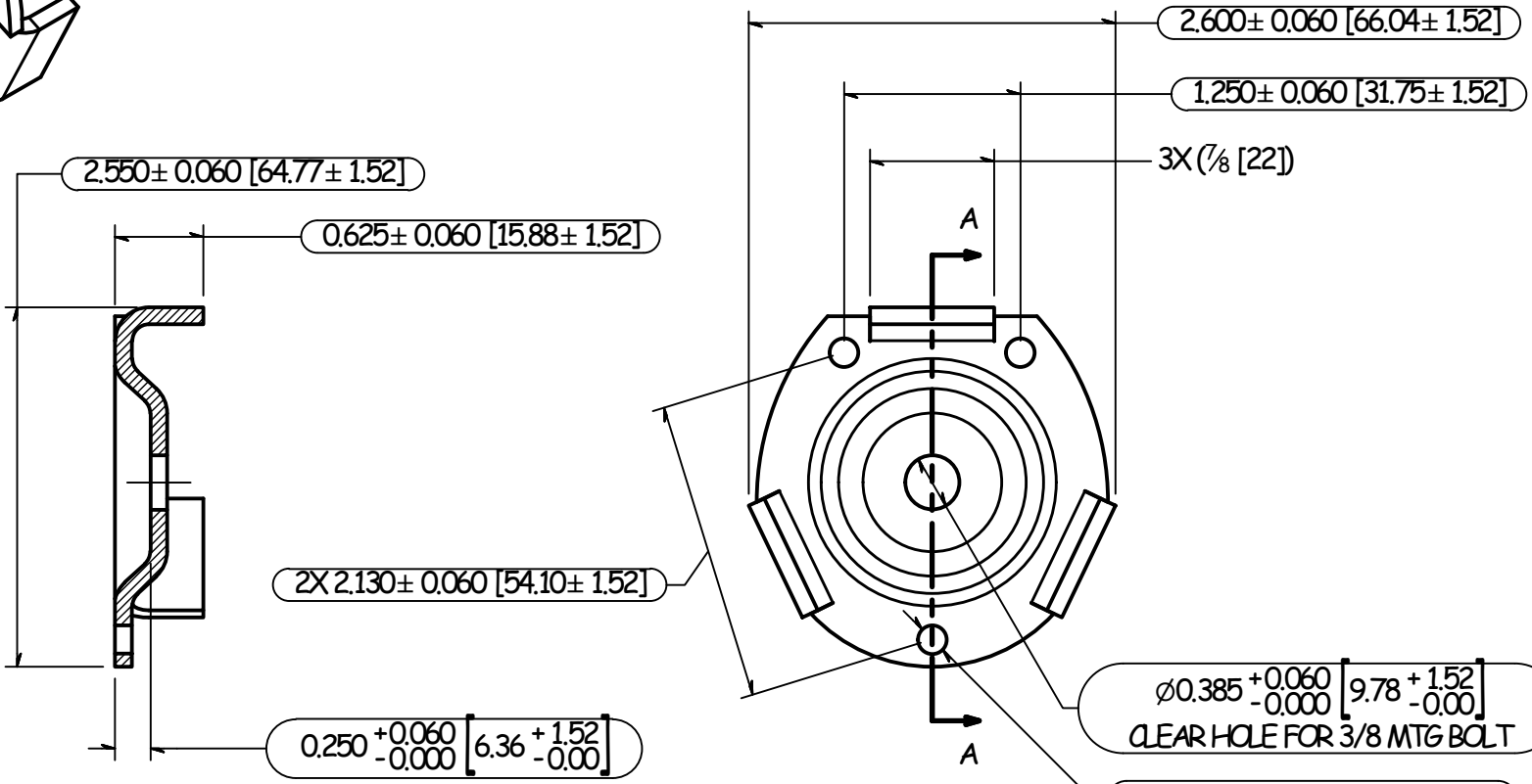
SECTION A-A
